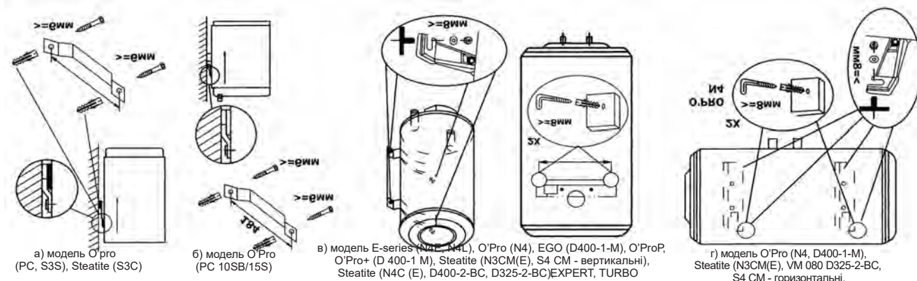
Рис. 4. Кріплення ЕВАД до стіни
